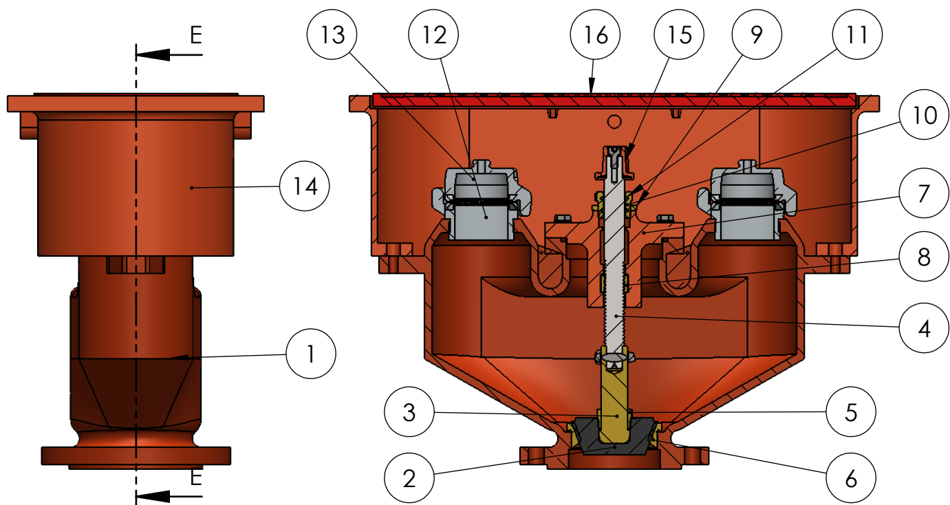
SECCIÓN E-E ESCALA 1 : 6
